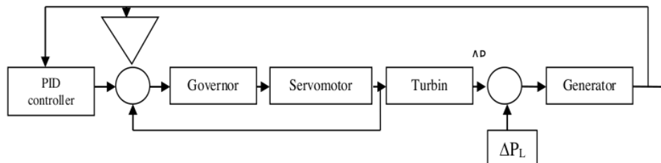
Gambar2. Pemodelan pembangkit Mikrohida [8]
