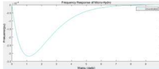
Gambar 4. Simulasi pembangkit mikrohidro tanpa kontrol
