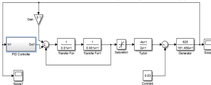
Gambar3. Pemodelan pembangkit Mikrohida [5]
