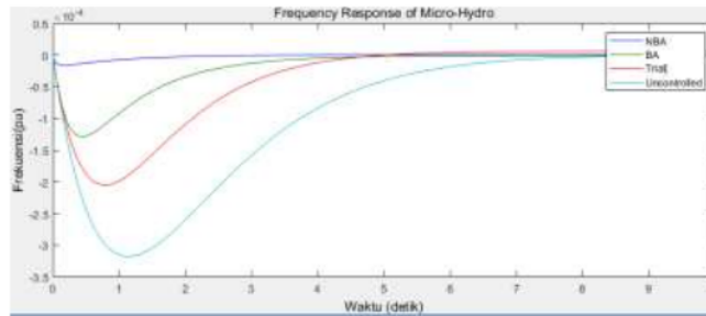
Gambar 7. Simulasi pembangkit mikrohidro PID-NBA
